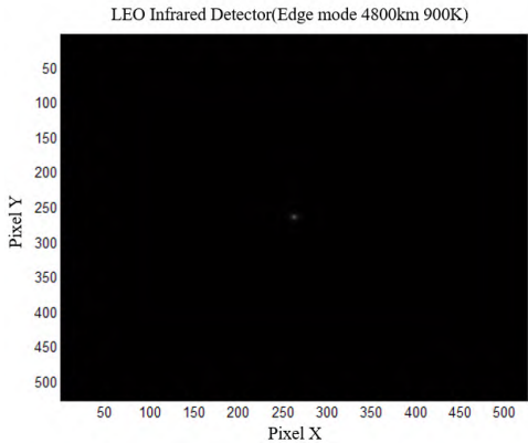
图14 临边模式下探测器焦平面模拟成像(900 K)
