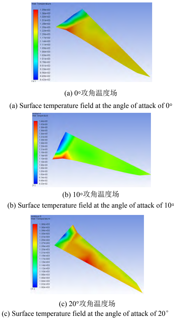
图4 CFD温度场仿真结果
