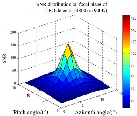
图15 临边模式焦平面像元信噪比分布(900 K)
