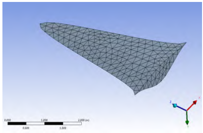
(b) 乘波体网格模型 (b) Grid model of wave-rider
