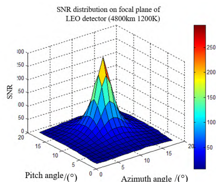
图13 临边模式焦平面像元信噪比分布(1200 K)
