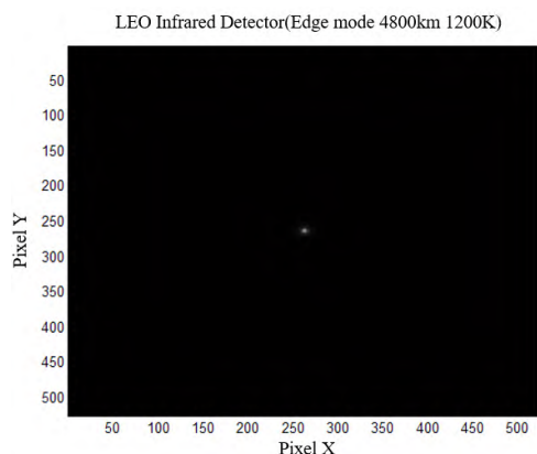
图12 临边模式下探测器焦平面模拟成像(1200 K)
