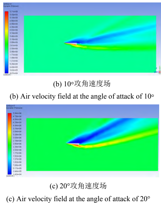
图3 CFD气动仿真结果
