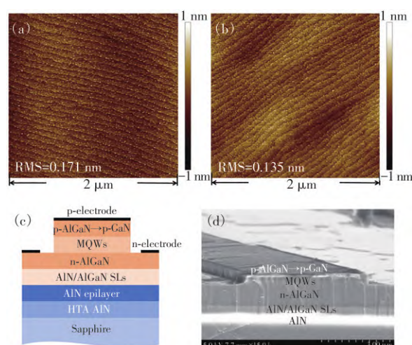
图 2 (a)在高温热处理 AlN 模板上外延生长 150 nm AlN 外延层后的表面 AFM 表征结果;(b)外延生长 AlGaIn/AlN 超晶格结构后 AFM 表面形貌表征结果;(c)LED 器件基本结构示意图;(d)LED 制备工艺探索过程中的 SEM 截面表征结果
