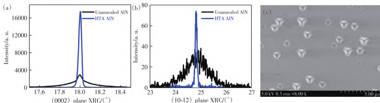
图1 (a)未热处理及高温热处理AlN模板的(0002)面XRC测试结果;(b)未热处理及高温热处理AlN模板的(10-12)面XRC测试结果;(c)熔融KOH/NaOH刻蚀高温热处理AlN模板表面位错刻蚀坑SEM表征结果
