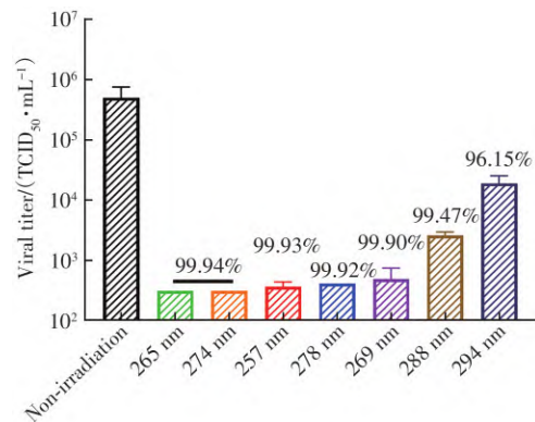
图4 不同波长 AlGaIn 基 LED 在本工作实验条件下的柯萨奇病毒灭活率
