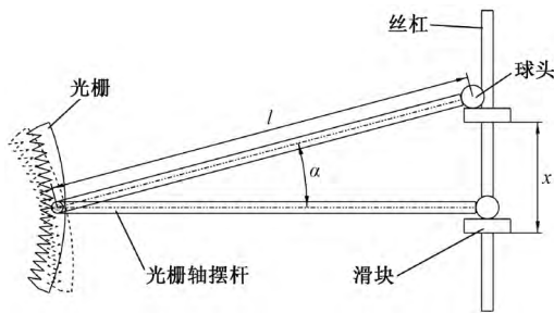
图3 凹面光栅单色仪驱动原理
