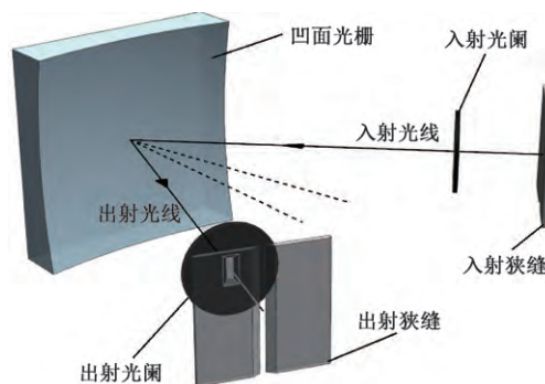
图2 单色仪分光部分工作原理图
