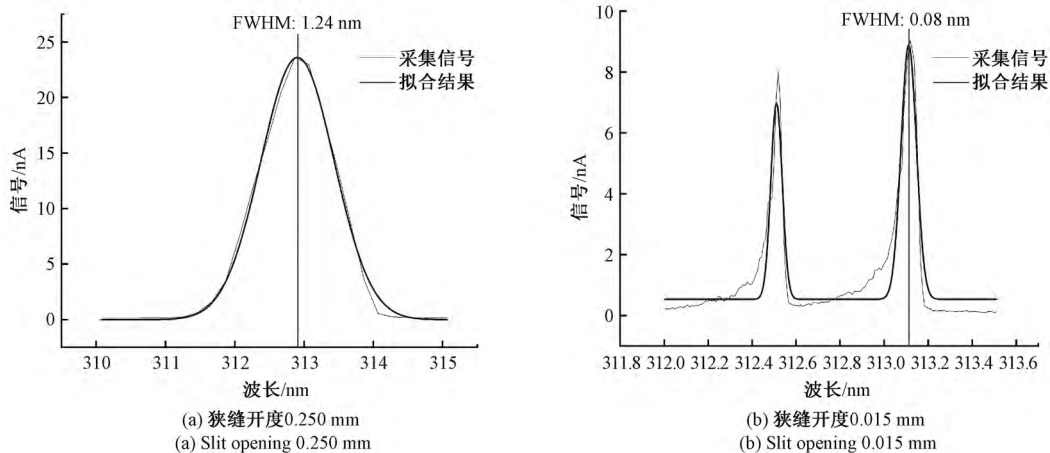
图 6 不同狭缝开度下的 313 nm 测试数据
