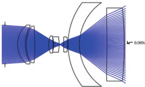
图 11 中心孔径光线追迹杂散光
