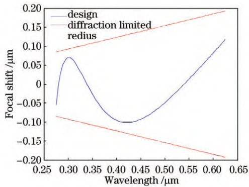
图 12 色焦移曲线
