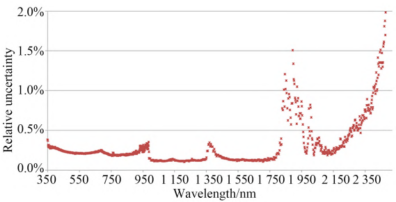
图 10 光谱测量模块的相对不确定度 Fig. 10 Relative uncertainty of spectral measurement module
