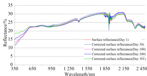
图 20 地表反射率校正
