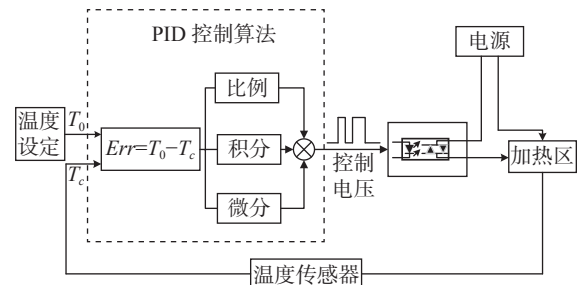
图 4 PID 控制原理图
