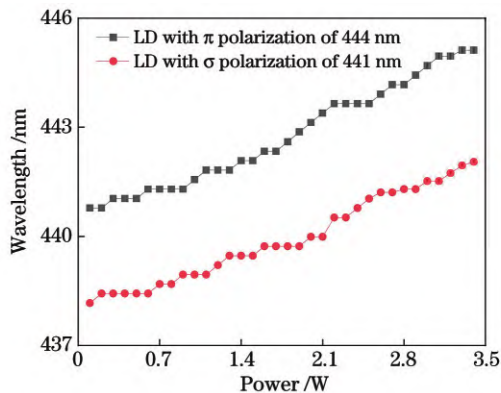
图 2 LD 波长随功率变化的曲线 Fig. 2 Curve of LD wavelength changing with power
