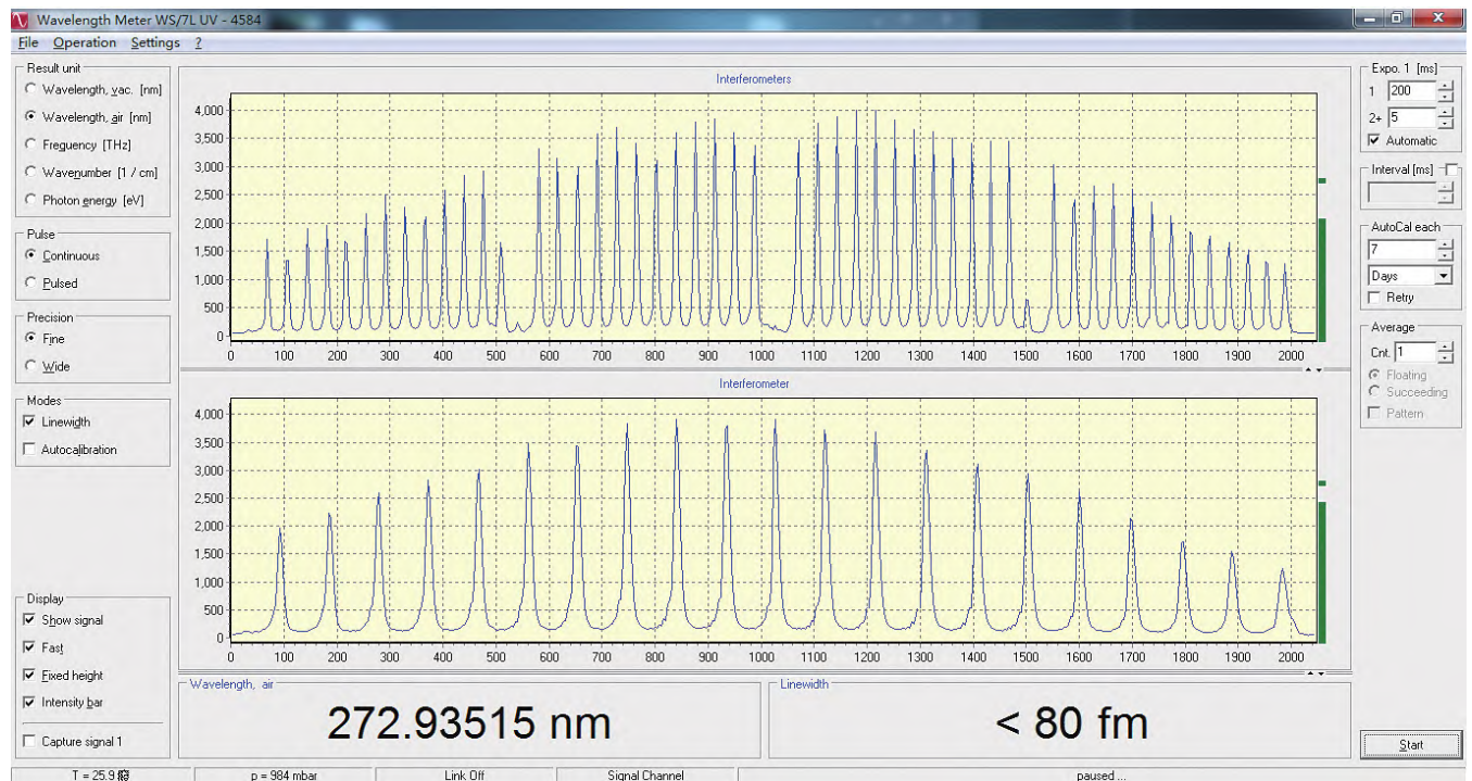
图 7 波长及线宽测试图 Fig. 7 Test diagram of wavelength and linewidth
