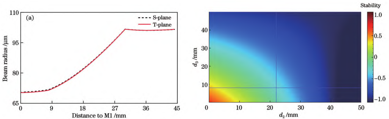
图 5 谐振腔分析。(a) 谐振腔内束腰半径模拟图; (b) 谐振腔稳定性模拟图
