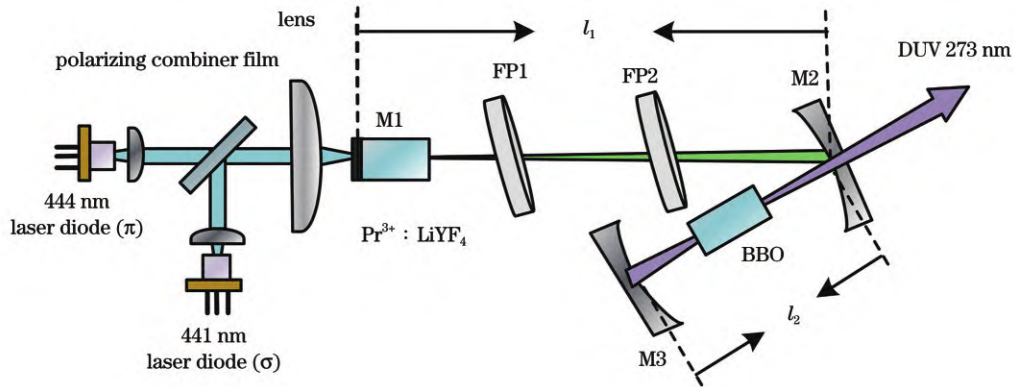
图 4 全固态单纵模 273 nm 深紫外激光器 Fig. 4 All solid state single longitudinal mode 273 nm DUV laser
