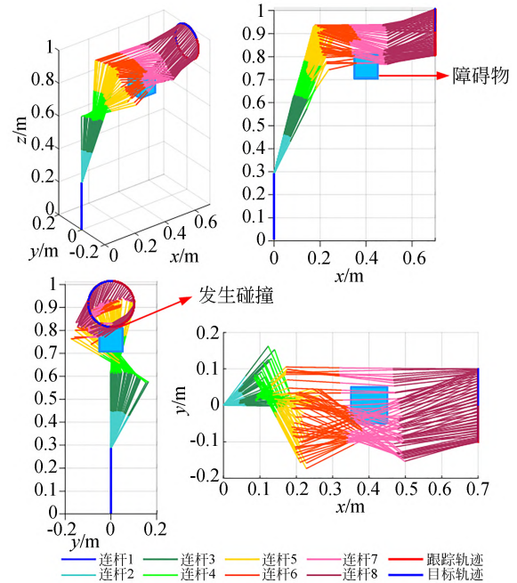
图4 关闭避障功能时的构型变化
