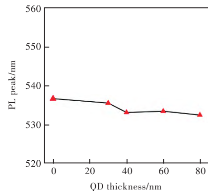
图3 不同CQD厚度的1DPC样品的PL峰值位置 Fig.3 PL peak position of 1DPC samples with different thickness of CQD
