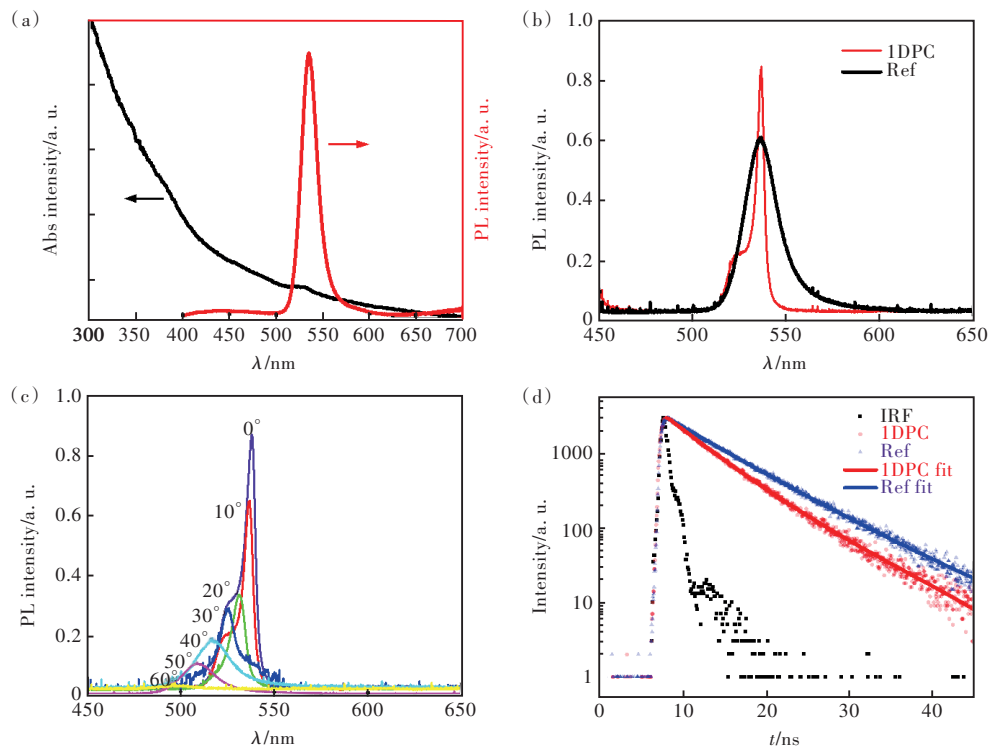
图2 1DPC样品的发光特性。(a)CQD薄膜的吸收和光致发光谱;(b)1DPC样品和参比样品的PL光谱;(c)1DPC样品的变角度PL光谱;(d)仪器响应函数以及1DPC样品和参比样品的荧光寿命。
