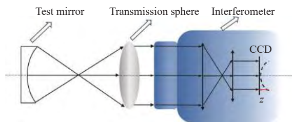
图 2 干涉仪检测球面台阶测试板光路模型
