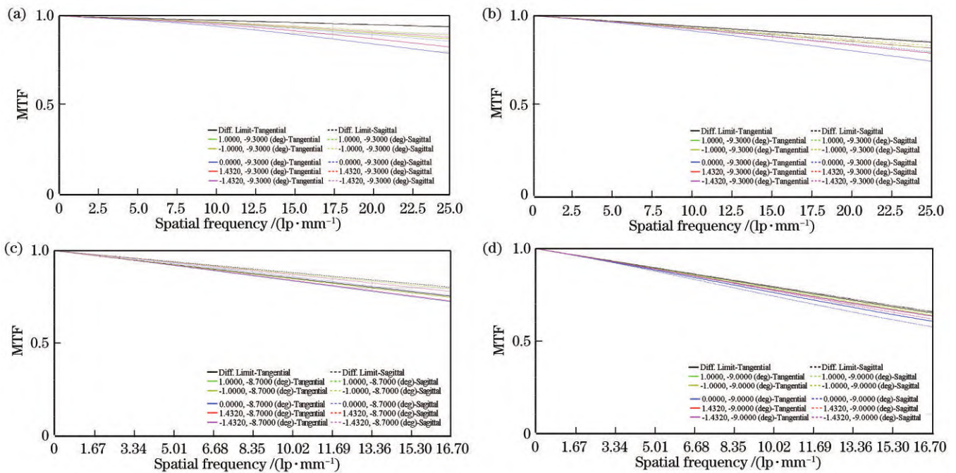
图 8 全系统各谱段中心波长处 MTF 曲线图。(a) 0.7 \mu\text{m} ; (b) 1.7 \mu\text{m} ; (c) 4.0 \mu\text{m} ; (d) 10.2 \mu\text{m}
