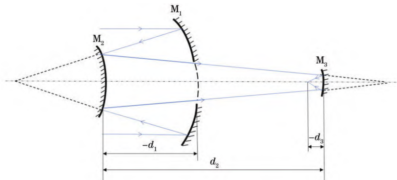
图 2 同轴三反结构
