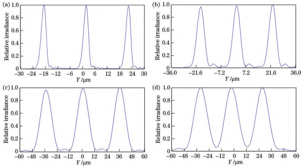
图9 各谱段点扩散函数截面图。(a) VNIR; (b) SWIR; (c) MWIR; (d) LWIR
