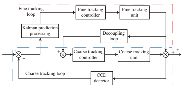
图 3 基于 Kalman 滤波的复合轴控制结构图
