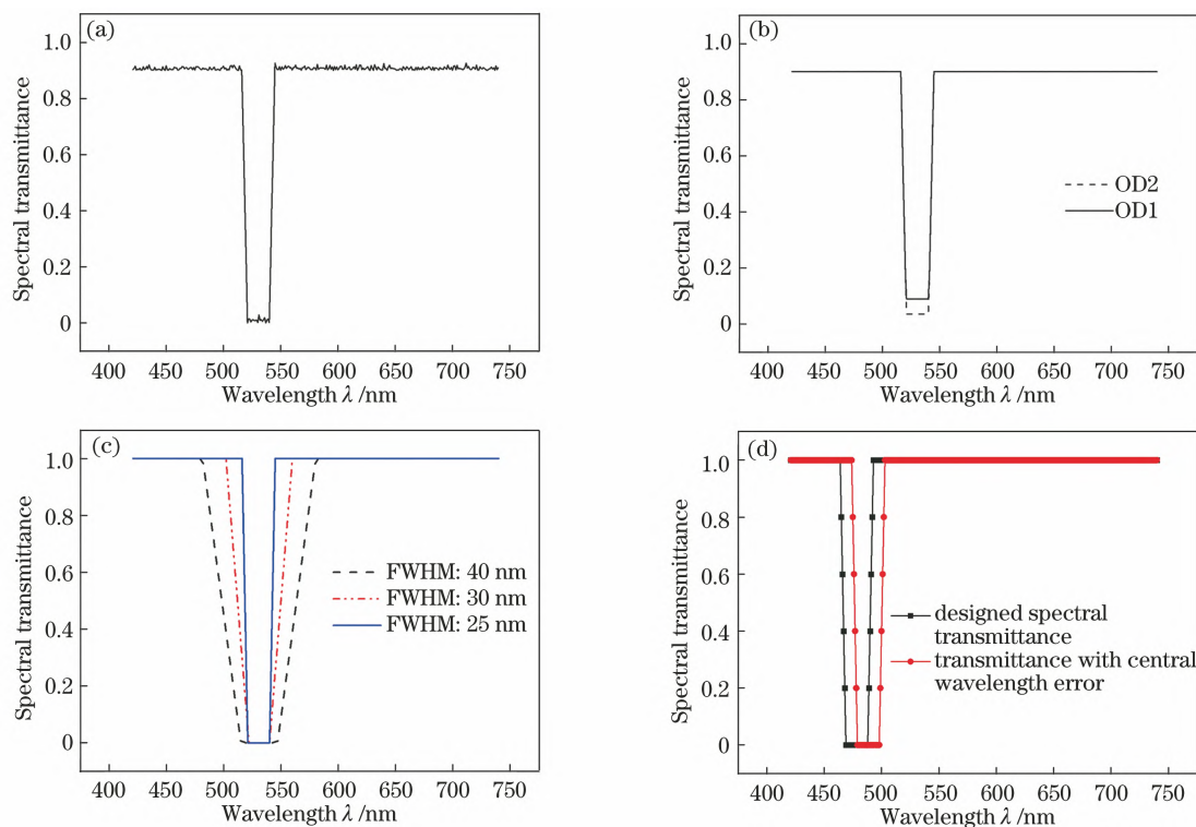
图 5 光谱透过率的主要误差类型。(a)全波段的随机误差;(b)截止波段的光密度误差;(c)带阻波段的半峰全宽误差;(d)带阻波段的中心波长位置偏差
