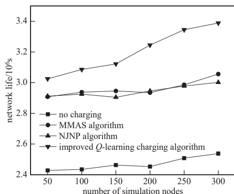
Fig.5 Network life comparison 图5 网络寿命比较图
