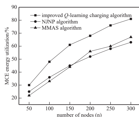
Fig.7 Energy utilization comparison 图7 能量利用率比较图
