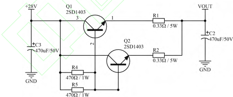
图 3. 两个三极管并联构成调整网络
