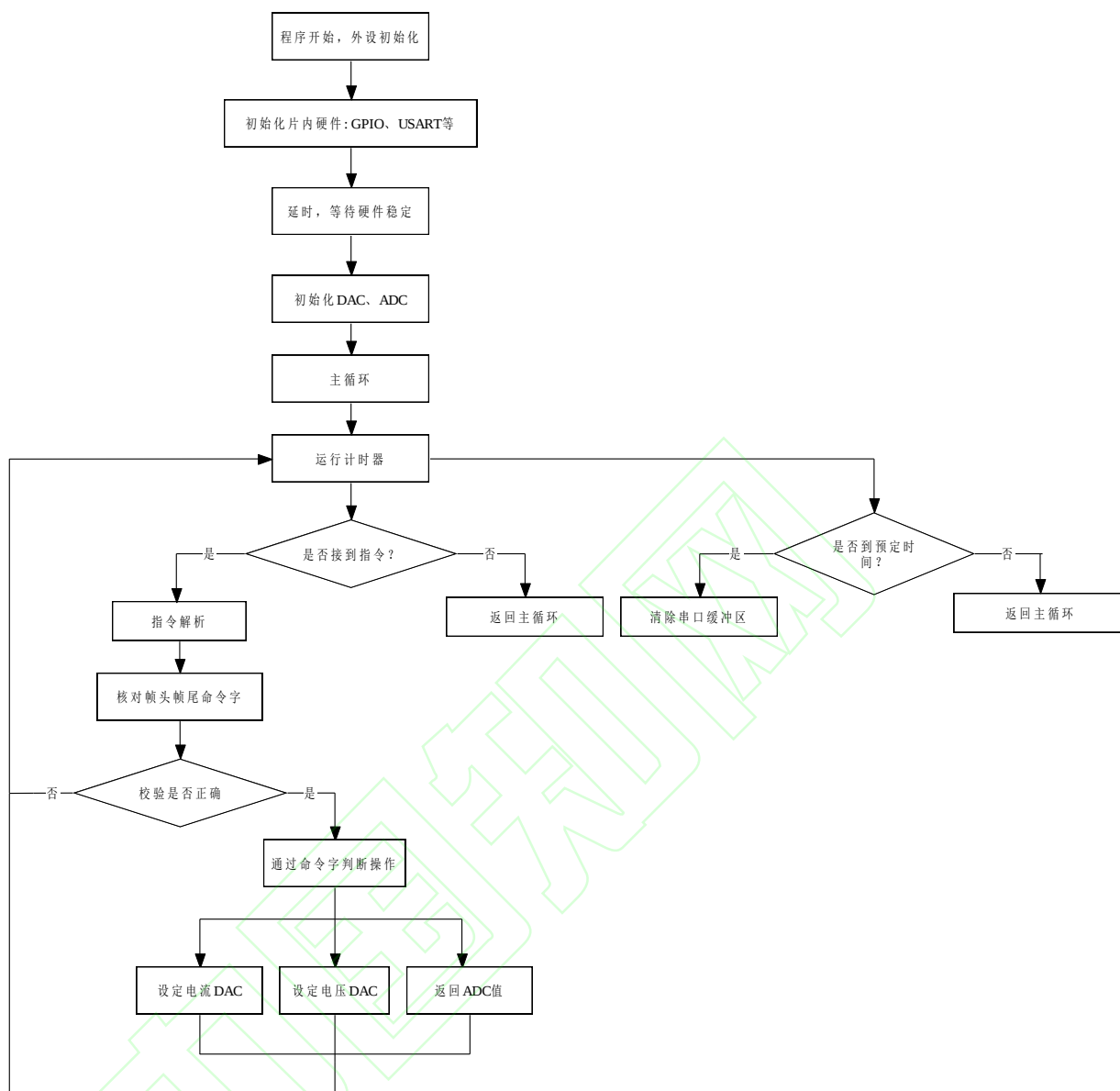
图 10. 程序流程图
