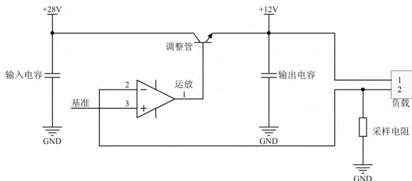
图 2. 恒流线性降压电路拓扑
