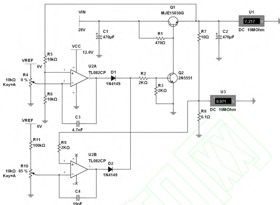
图 7. Multisim 仿真图
