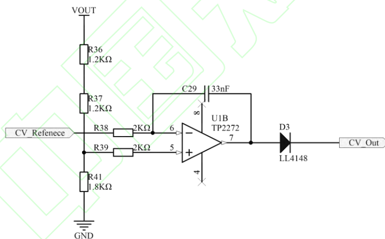
图 5. 恒压闭环电路
