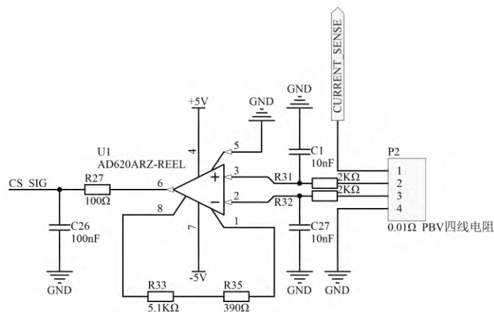
图 4. PBV 四线电阻检流电路
