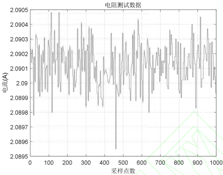
图 11. 电阻负载恒流数据
