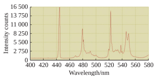
图2 Pr:YLF 晶体的荧光谱线 Fig. 2 Emission spectra of Pr:YLF crystal
