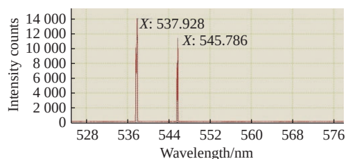
图3 基频光光谱测试图 Fig. 3 Spectrogram of fundamental laser
