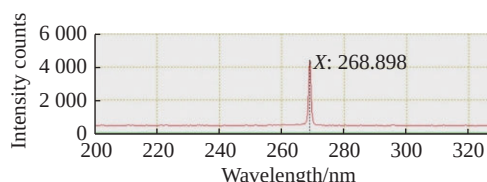
图 4 连续紫外光光谱测试图
