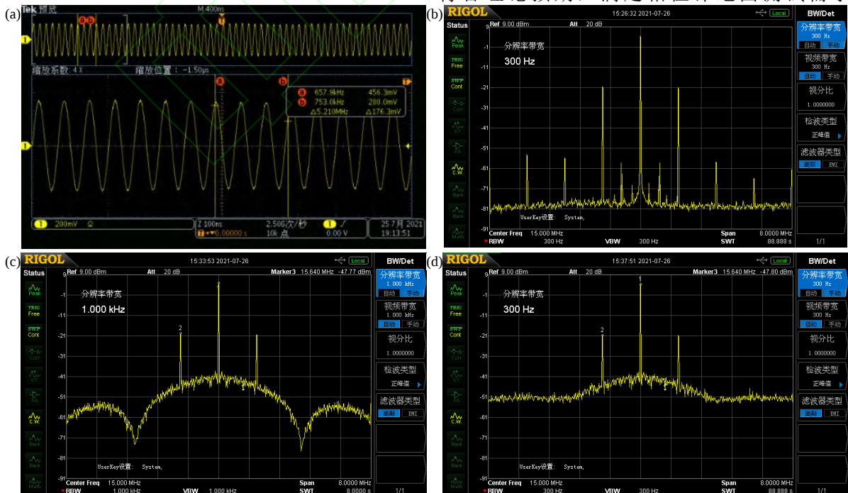
图 9 (a)主载波拍频与两个时钟边频耦合信号的波形图;(b) 主载波拍频与两个边时钟频耦合信号的频域图;
