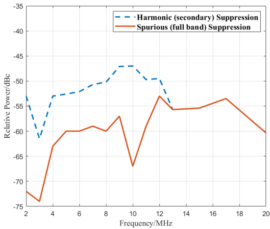
图 8 2~20 MHz 频段内谐波抑制程度示意图
