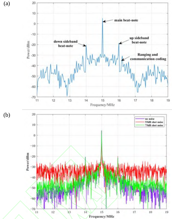
图 7 (a)主体信号的频谱图;(b)耦合散粒噪声的主体信号的频谱图
