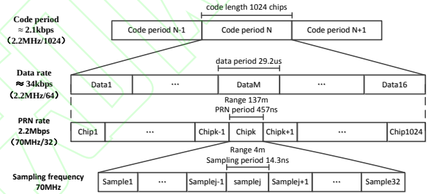
图 2 测距通信系统的设计参数
