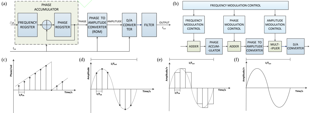
图3 (a) 直接数字合成器基本原理结构图；(b) 带调制功能的直接数字合成器原理框图；
