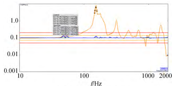
(a) 未安装金属橡胶减振器
