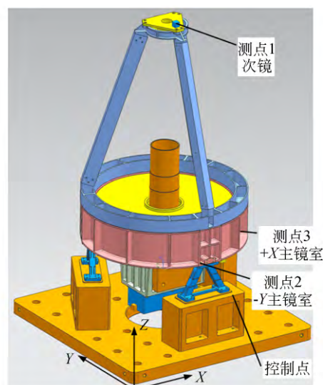
图12 振动测试点
