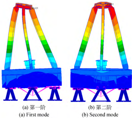
图 9 空间相机前两阶模态振型
