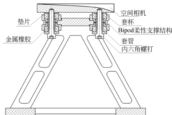
(b) 金属橡胶减振器剖视图
