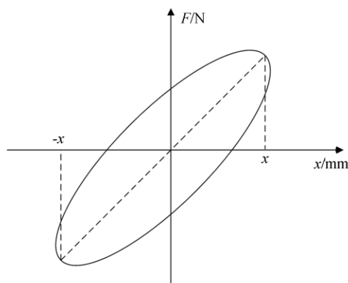
图1 金属橡胶的迟滞曲线
