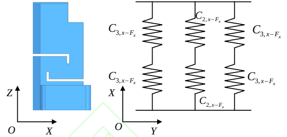
图 7 柔性支撑座在 X 方向上的等效力模型
