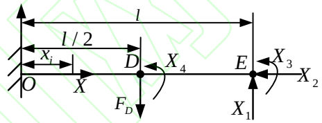
(c) 等效静定结构模型
