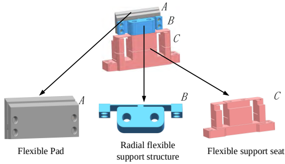
图 3 柔性支撑组件及其各部分结构件
