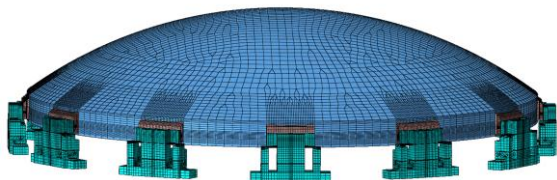
图 11 网格划分图
