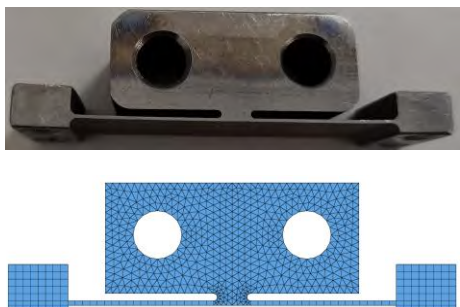
图 9 径向柔性支撑结构及其有限元模型
