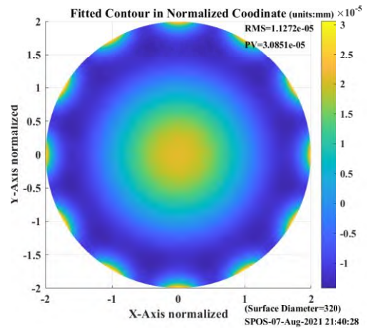
图 15 镜面上表面面形云图
