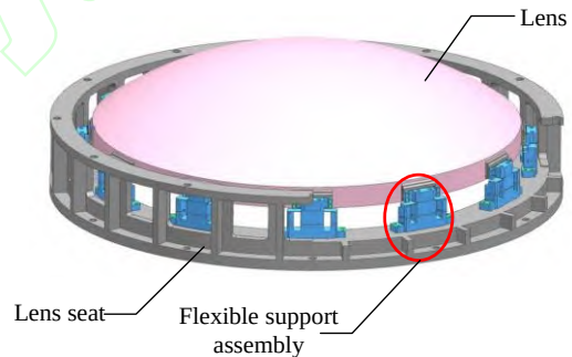
图 2 透镜组件整体结构示意图
