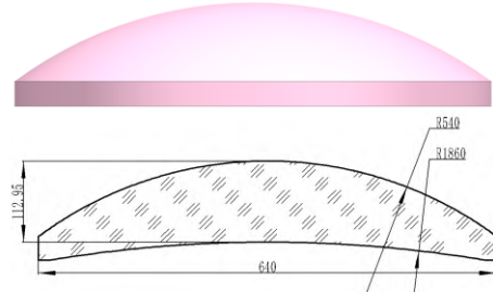
图 1 透镜形状及尺寸参数
