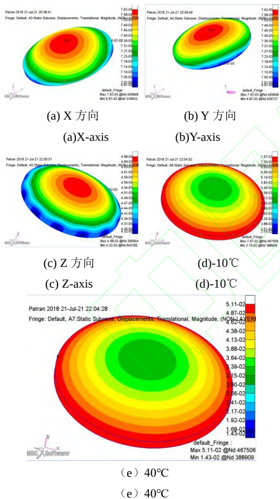
图12 各工况下仿真结果
