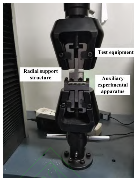
图 10 实验测试装置
