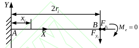
图 5 柔性铰链受力分析示意图
