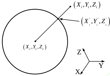
图 14 球面数据拟合原理示意图
