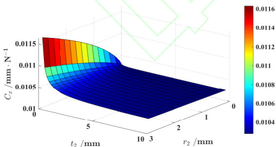
(b) 柔性度 C_x 随设计参数 t_2 和 r_2 的变化关系 (b) The relationship between flexibility C_x and design parameters t_2 and r_2
