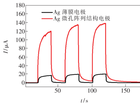
图8 MgZnO 紫外探测器在 10 V 偏压下电流随周期性开关 254 nm 波长紫外光的变化曲线
