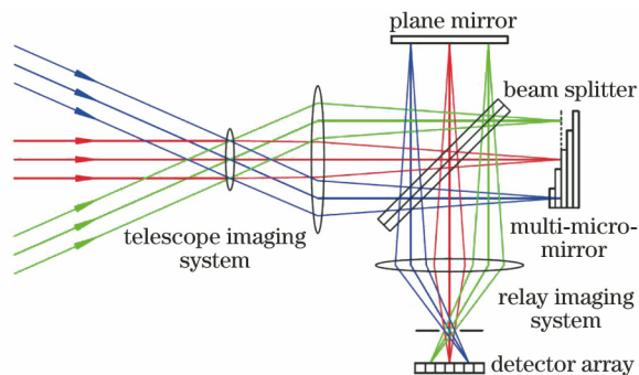
图1 像场调制傅里叶变换成像光谱仪的原理图
