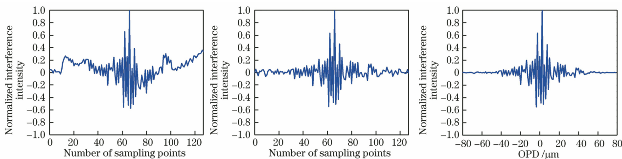
图 13 干涉图序列的数据处理。(a)提取;(b)基线校正;(c)寻址切趾
