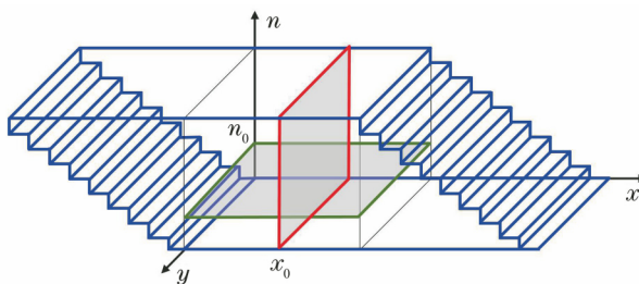
图2 像场调制傅里叶变换成像光谱仪的数据结构
