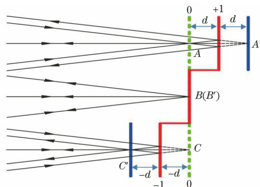
图 3 多级微反射镜对像场的光程调制过程图示
