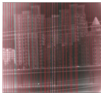
图 9 边缘检测与插值拟合后的图像剪切线
