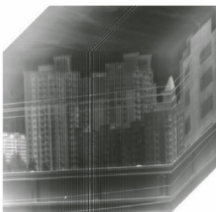
图 8 干涉图像数据立方体
