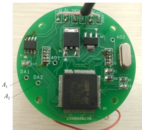
图6 角位移监测系统电路
