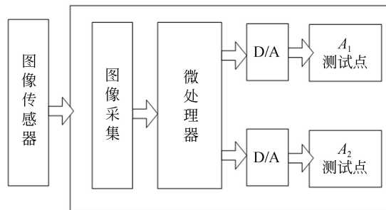
图5 角位移监测系统原理
