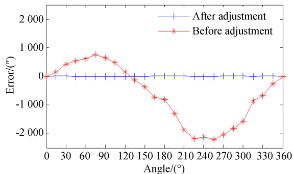
图11 偏心调节前后的测角误差对比
