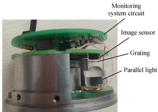
图 7 角位移测量实验装置
