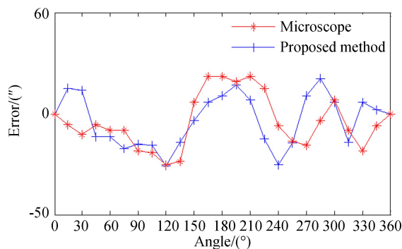
图12 不同偏心调节方法的测角误差对比
