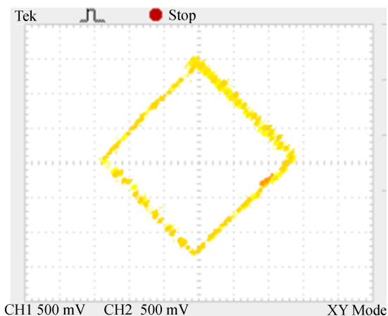
图 9 精确调节后的监测信号
