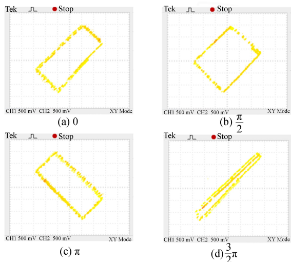
图 8 四个位置处的监测信号波形
