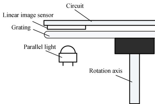
图 1 图像式角位移测量系统光路
