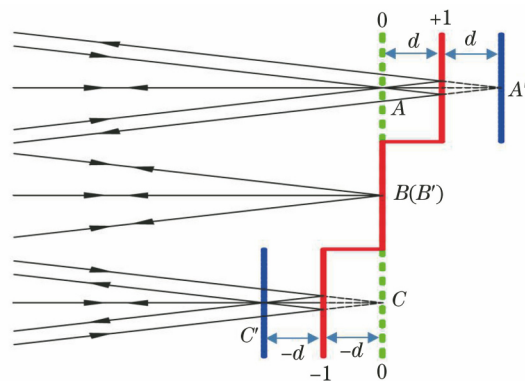
图 3 多级微反射镜对像场的光程调制过程图示
