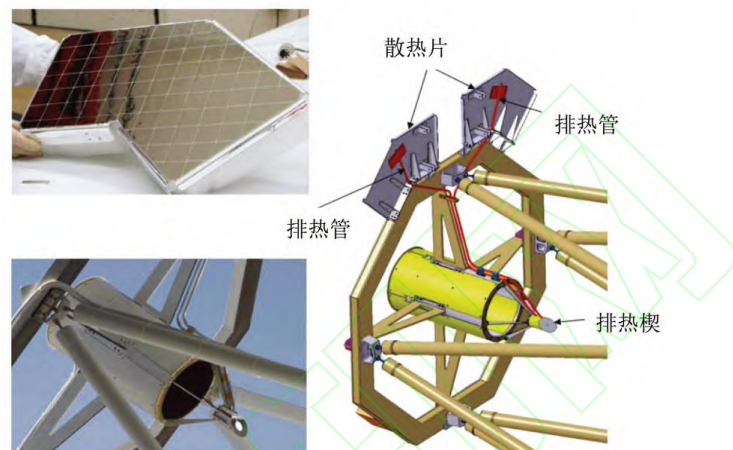
图 3 副镜及前环组件 [20] 。焦点 F1 处安装了一个排热楔。其中心的小圆孔只允许一部分光透过并到达副镜 M2 处，形成视场光阑。排热楔的表面涂层一方面可以反射 99% 的入射光，一方面吸收一小部分能量并通过排热管送到散热片。这样可以保持排热楔的温度在 25 °C 以下。
