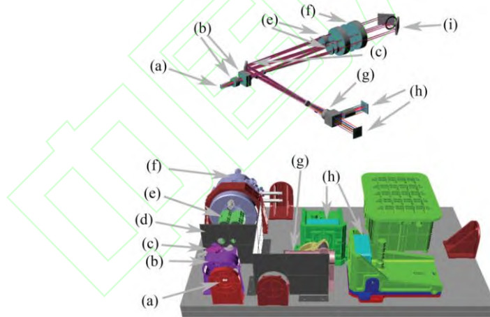
图 6 磁像仪光路图(上)和对应的三维结构图(下) [22] 。为了便于理解，图中用字母将光路和三维结构中对应的仪器标注了起来。在光路图中，(a)F4；(b)前置滤光器、两个延迟器；(c)45°镜；(d)灰色挡板；(e)准直镜；(f)F-P 干涉仪；(i)45°镜和孔径光阑；(g)前后两个透镜、分束器。(h)CCD 终端。光路的三维结构图，F4 被棕红色的装置封装(a)，用于光束通过；(b)是安装有前置滤光器和两个延迟器的紫色装置；(c)鲜红色装置的 45°镜；(d)遮挡杂散光的灰色挡板。挡板上有两个小孔。(e)绿色装置的准直镜；(f)安装在银灰色热稳定外壳里的 F-P 干涉仪；(i)两个 45°镜；(g)粉红色的分束器；(h) CCD。
