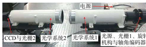
图4 实验设备布局
