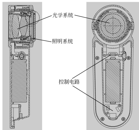
图 9 总体机械图
