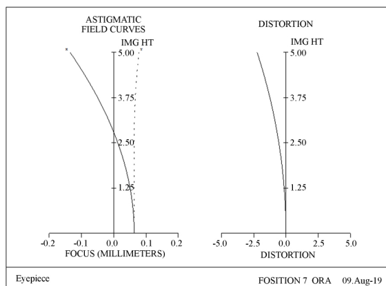
图 5 偏振皮肤镜场曲和畸变曲线
