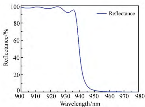
图 2 二色分光镜的膜系曲线
