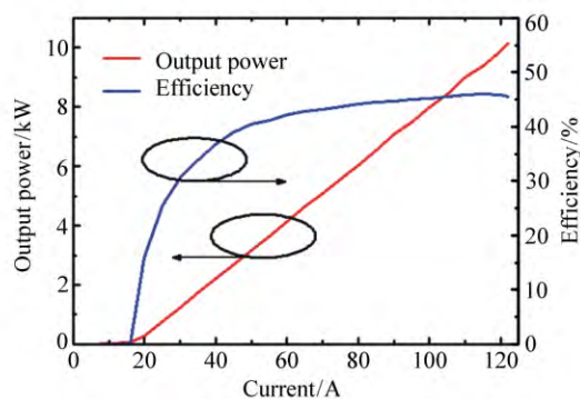
图7 功率和效率随电流的变化曲线
