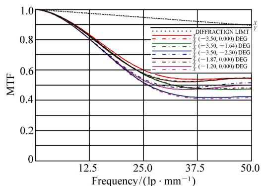
图6 系统MTF曲线图
