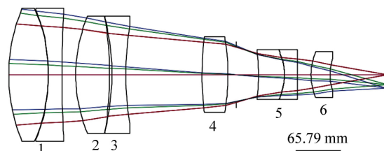
图3 单组物镜二维轮廓图
