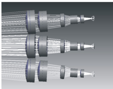
图4 多角度耦合四分幅光学系统结构主视图
