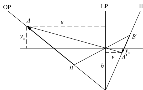
图 2 沙姆定律几何证明
