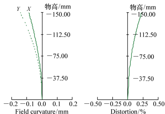
图7 场曲和畸变性能
