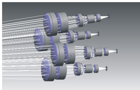
图5 多角度耦合四分幅光学系统结构立体视图
