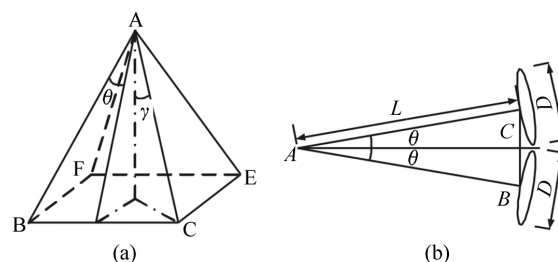
图 1 (a) 物点与 4 个系统的立体结构; (b) 相邻两个系统的几何关系
