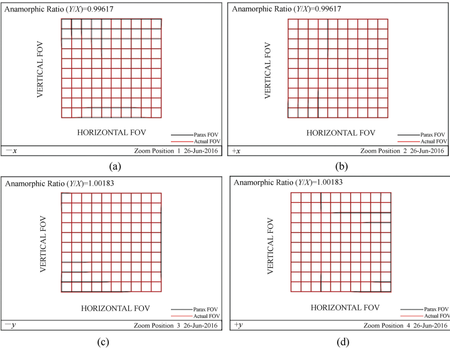
图 8 ( a ) 、( b ) 、( c ) 和 ( d ) 分别为结构 1、2、3 和 4 的畸变网格图 Fig. 8 ( a ) , ( b ) , ( c ) and ( d ) are the distortion grid figures of configuration 1 , 2 , 3 and 4 respectively
