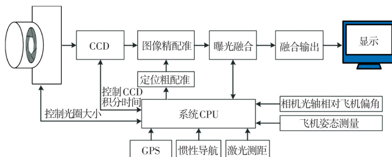
图1 航空相机多曝光融合系统结构图
