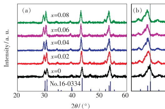
图 3 (a) Na_{1-x}K_xErF_4@NaLuF_4 ( x: 0 \sim 8\% ) 掺杂不同浓度 K^+ 的纳米晶体的 XRD 衍射图谱及标准六角相 JCPDS No. 16-0334 图谱; (b) XRD 图谱在 53.4^\circ 处放大的衍射峰。
