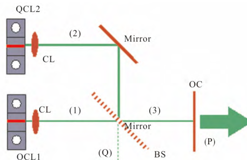
图 1 量子级联激光器迈克尔逊腔相干合束示意图 [17]
