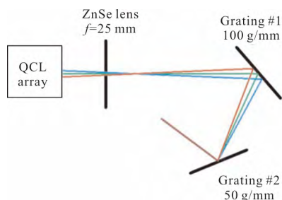
图 5 量子级联激光器双光栅光谱合束示意图 [26]
