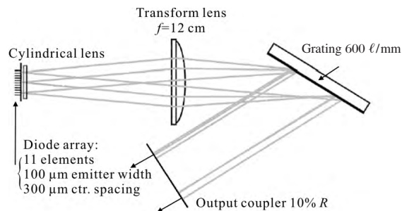
图 3 碲化物量子阱激光器线阵光谱合束示意图 [20]
