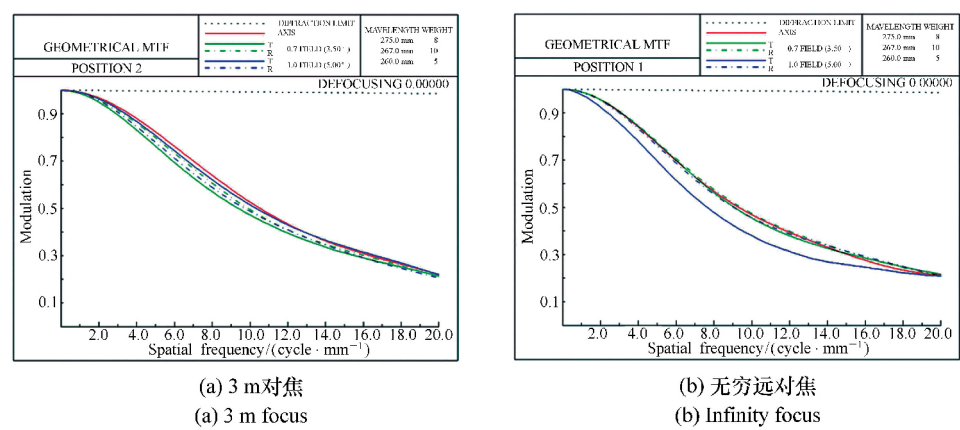
图 3 传递函数曲线 Fig. 3 MTF curve
