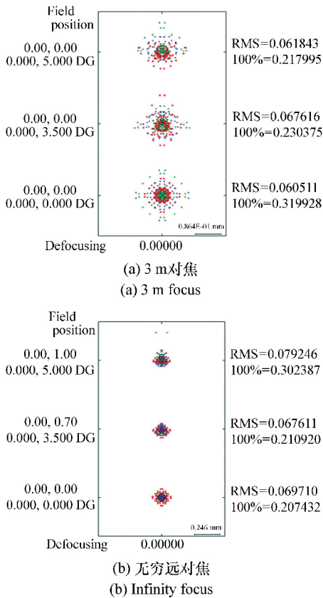
图 2 点列图 Fig.2 Spot diagram
