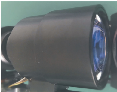
图 4 紫外光学系统实物图 Fig.4 Ultraviolet optical system
