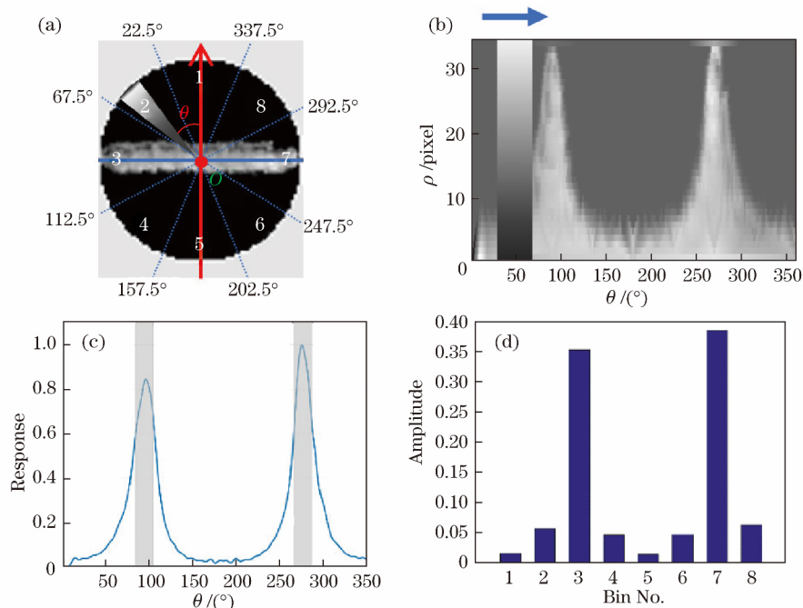
图 6 目标切片的灰度分布特征。(a) 方向和区域划分示意图；(b) 极坐标系内的图像；(c) 灰度分布曲线；(d) 灰度分布直方图
