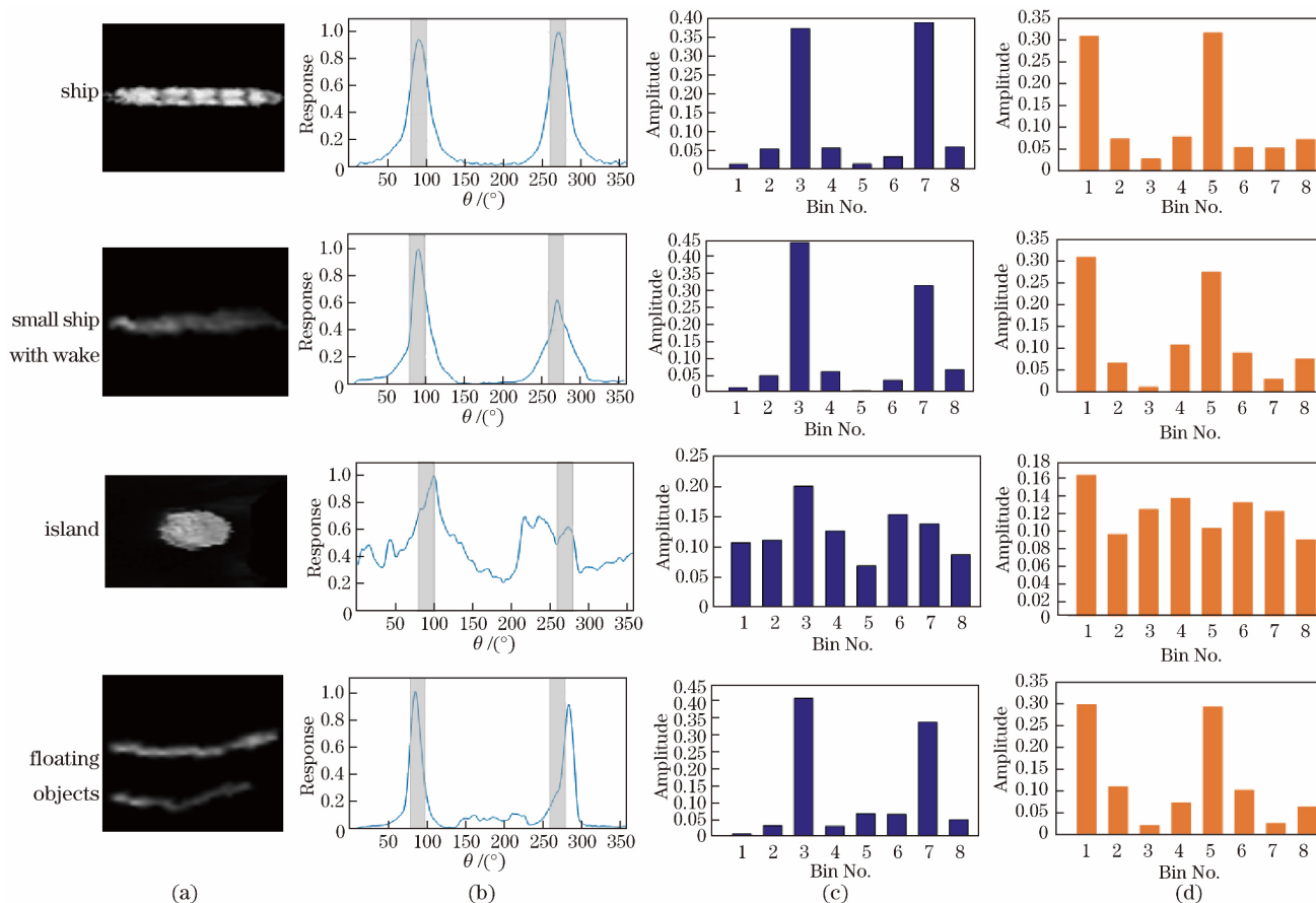
图 8 目标切片的几何特征描述。(a) 预处理后的目标切片;(b) 灰度分布曲线;(c) 灰度分布直方图;(d) 梯度方向直方图 Fig. 8 Geometric characterization of target chips. (a) Prescreened target chips; (b) grayscale distribution curve; (c) grayscale distribution histogram; (d) gradient oriented histogram
