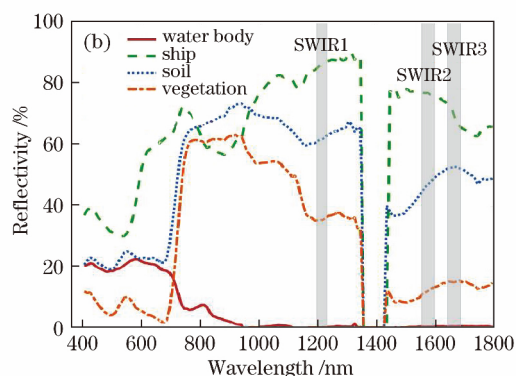
图 2 (a) 场景图像; (b) 典型地物反射率曲线
