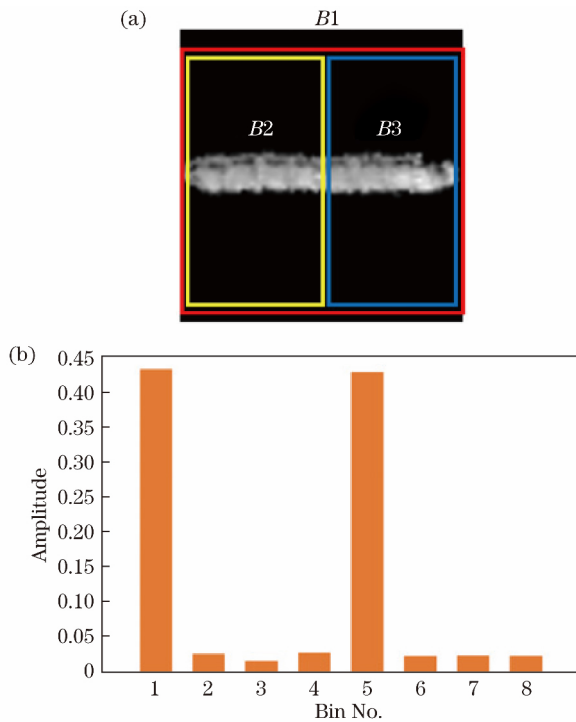
图 7 S-HOG 描述子。(a) S-HOG 描述子的区域划分; (b)图 7(a)中 B1 区域的梯度方向直方图
