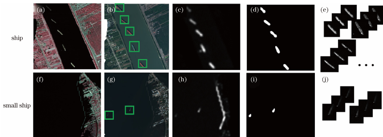
图 4 显著性检测及目标切片提取。(a)(f) SWIR 输入图像; (b)(g) 同一场景的可见光图像(手工标记出目标);
