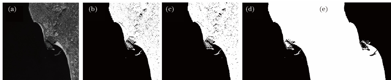
图 3 (a)强度图 I ; (b)对比度拉伸图 I' ; (c)陆地掩模; (d)填补孔洞后的陆地掩模; (e)水体掩模
