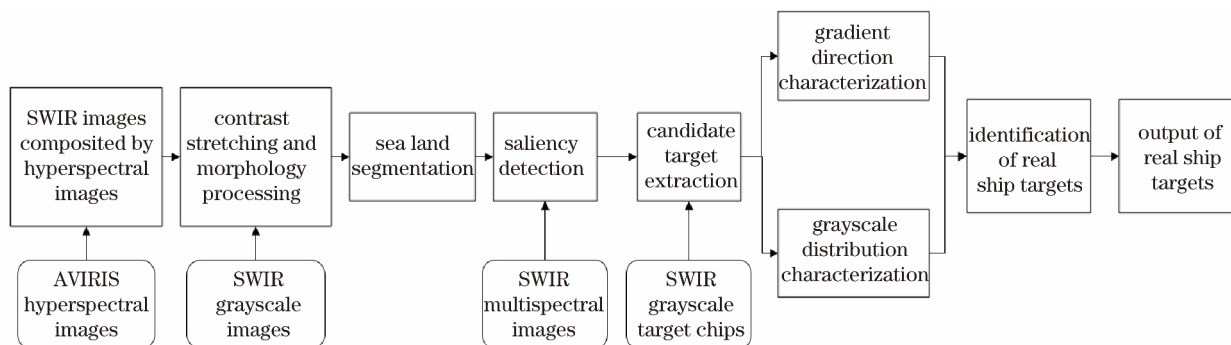
图 1 基于 SWIR 影像的船只自动检测方法的流程
