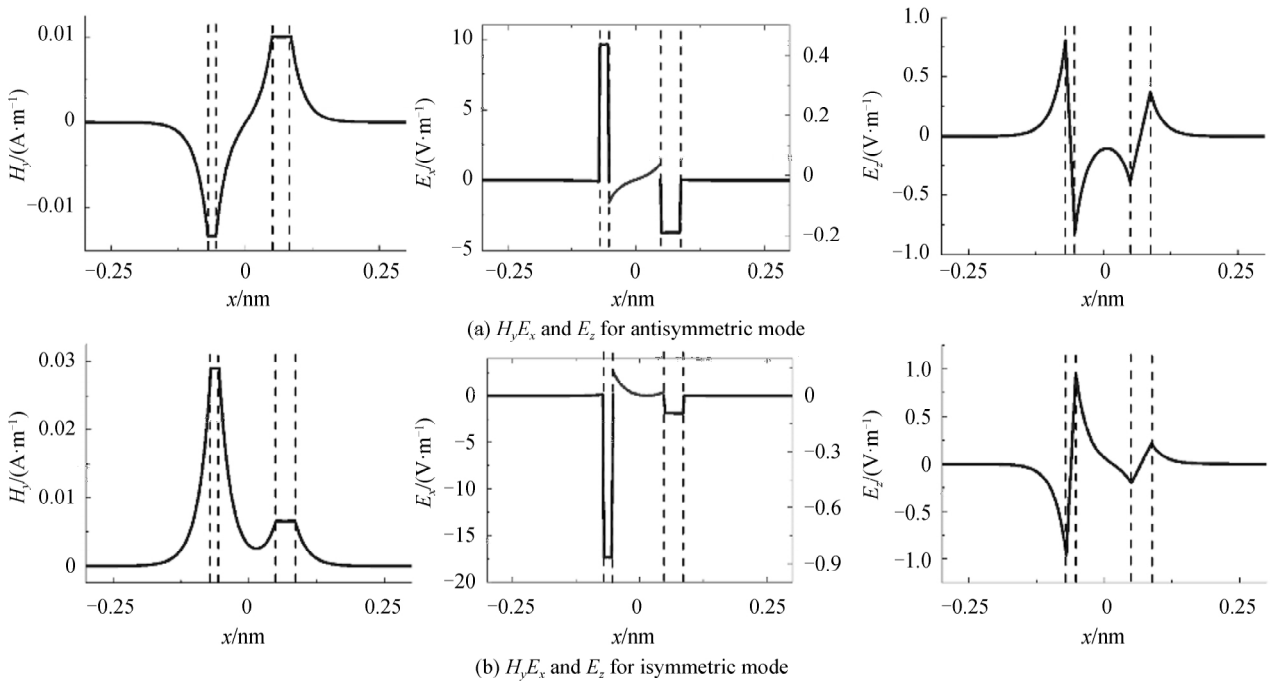
图4 双缝结构的横向平分线上电磁场分量的分布曲线(垂直虚线标定狭缝边界)
