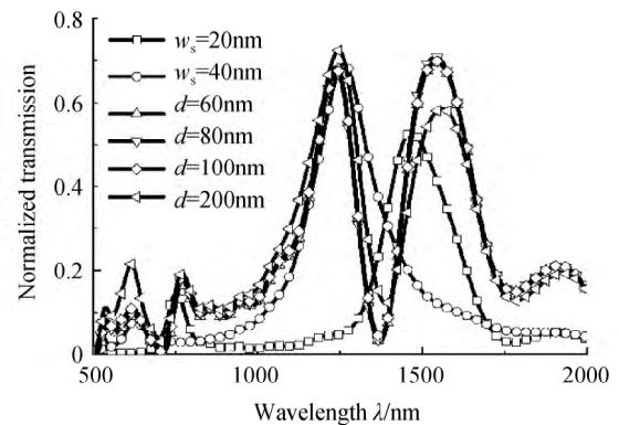
图 2 双缝结构在不同金属隔层下的透射谱
