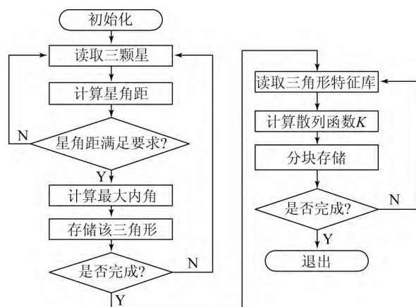
图 2 导航三角形构建流程
