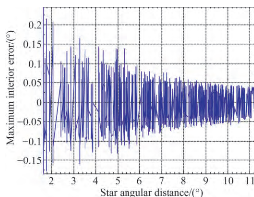
图 4 星角距对内角精度的影响
