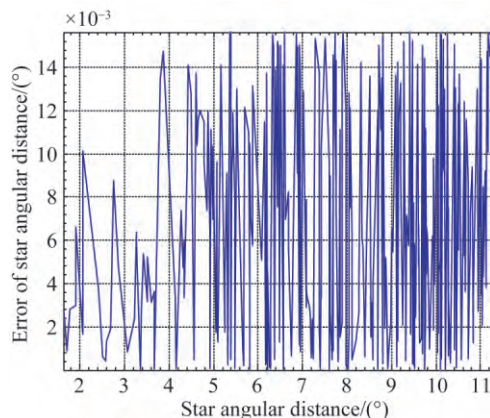
图 3 星点定位误差对星角距测量精度的影响
