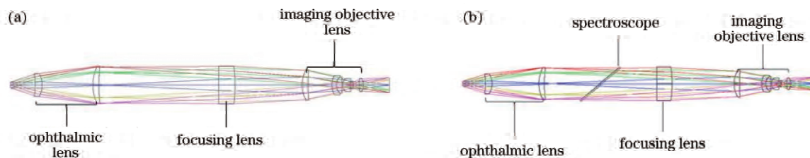
图 5 成像系统初始结构。(a)未加分光镜;(b)加入分光镜
