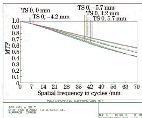
图 7 成像系统的 MTF 曲线
