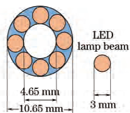
图 12 环形光源示意图
