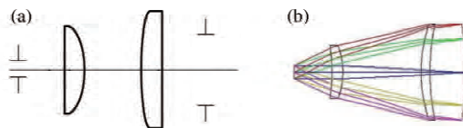
图 4 接目物镜结构。(a)原型;(b)优化结果
