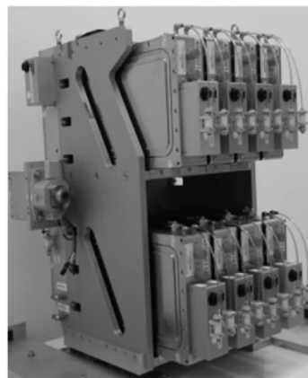
图 9 Teradiode 的 8\text{ kW} 直接半导体激光器结构图
