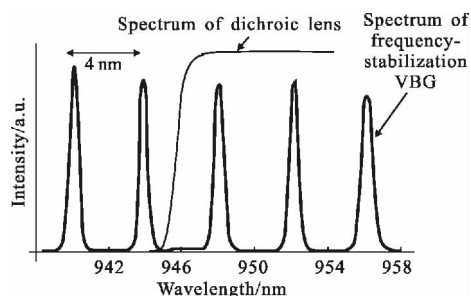
图 6 Direct photonics 实现间隔 4\text{ nm} 的 5 波长合束光谱分布
