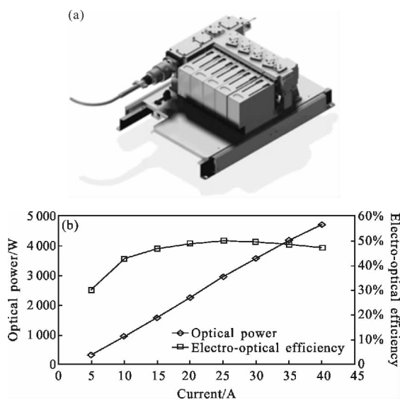
图 4 Dilas 研制的 4 kW、400 \mu\text{m}/0.12 光纤输出半导体激光合束光源
