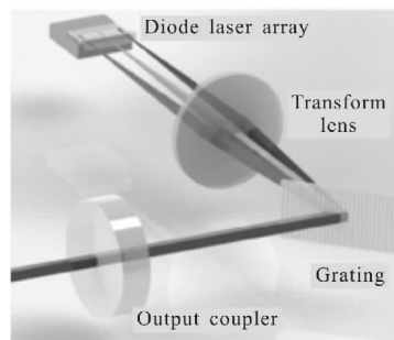
图 8 光谱合束原理
