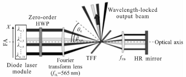
图 11 基于窄带滤光片的外腔反馈波长锁定结构
