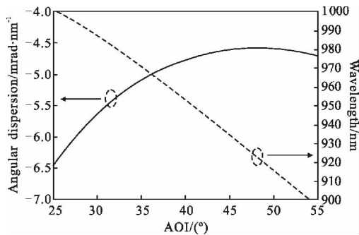
图 10 窄带滤光片的角度-色散-波长特性
