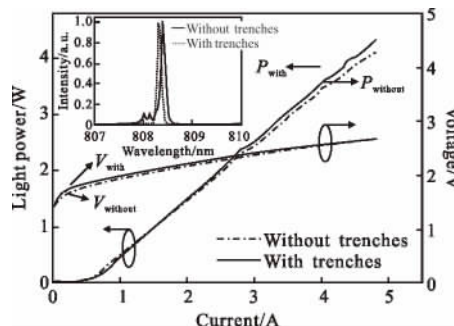
图 14 鱼骨形结构与不带鱼骨形结构激光器的 L-I-V 曲线
