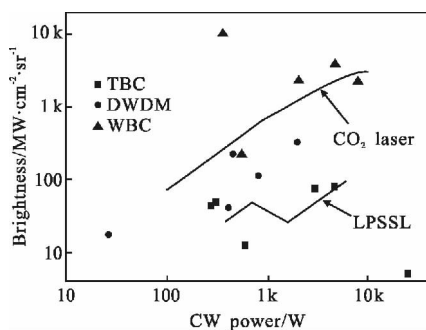
图 12 半导体激光源的功率-亮度分布及与其他类型激光器对比
