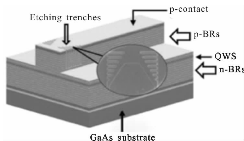
图 13 鱼骨形光子晶体结构激光器示意图
