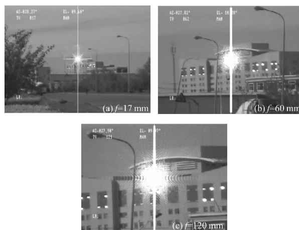
图 9 变焦光学系统的激光干扰仿真结果
