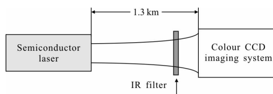
图 5 实验原理示意图
