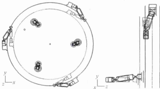
图 4 温度升高时的柔性支撑结构的变形
