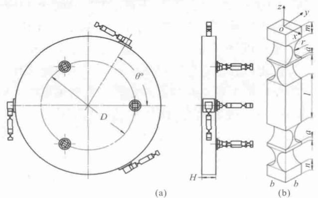
图 3 反射镜组件结构图
