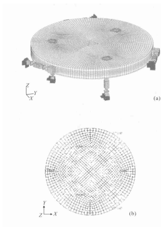
图 6 实体和参数化片体有限元模型
