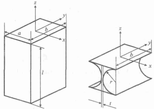
图 5 梁单元和圆切口柔性单元
