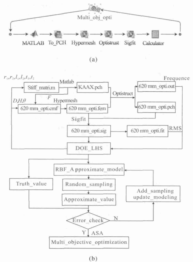
图 7 主镜组件多目标优化流程图
