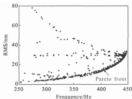
图 8 Pareto front 最优解集
