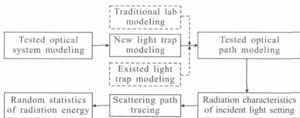
图 8 仿真实验流程
