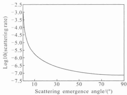
图 3 物化处理后材料表面的 BRDF 曲线
