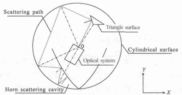
图 7 文中研制光陷阱的工作原理
