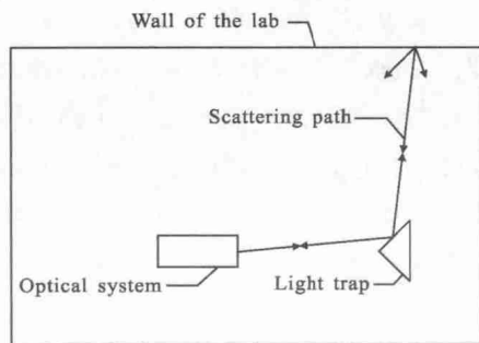
图 4 XMM 光陷阱中散射路径示意图
