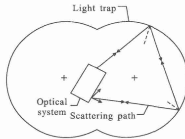
图 5 BALL 公司光陷阱中散射路径示意图
