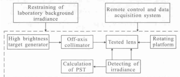
图 1 PST 测试系统组成示意
