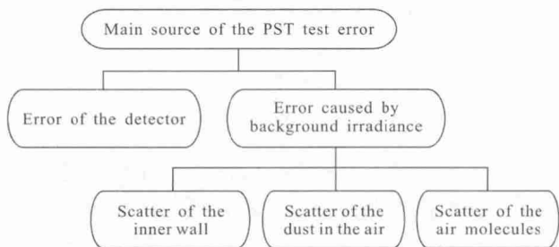
图 2 PST 测试的主要误差来源
