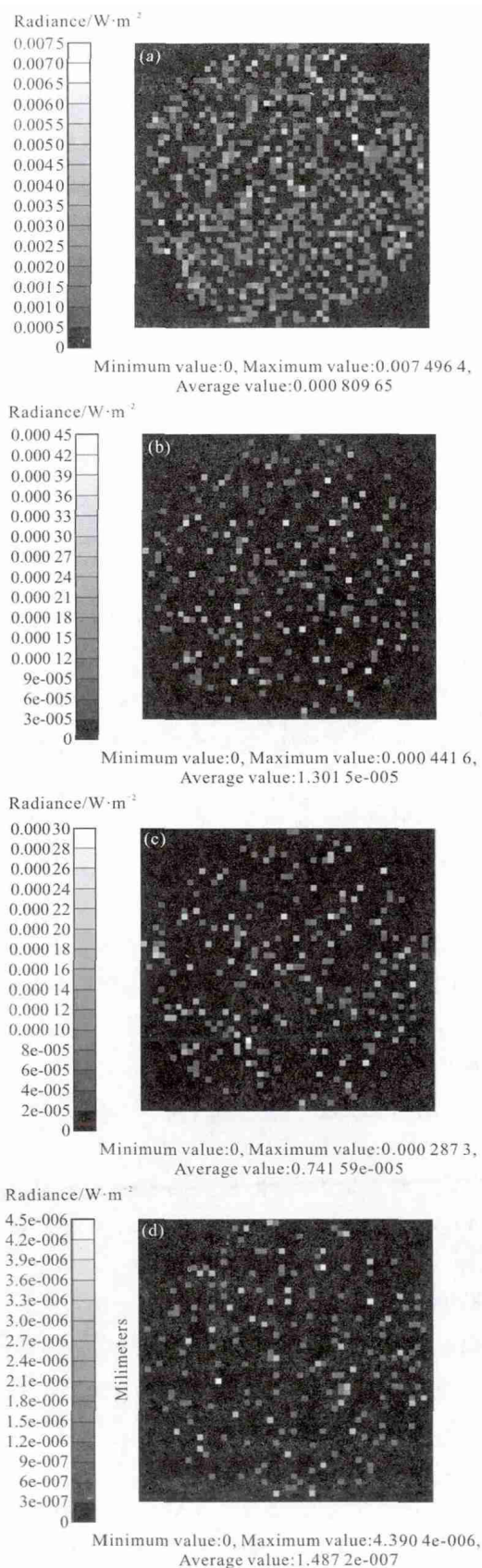
图 9 各光陷阱模型的仿真结果
