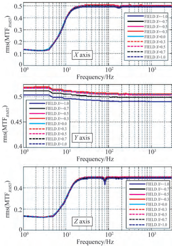
图 10 均方根 MTF_{RMS} 的频率响应 Fig. 10 Frequency response of MTF_{RMS}
