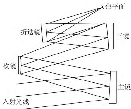
图 1 大口径空间相机光学系统示意图
