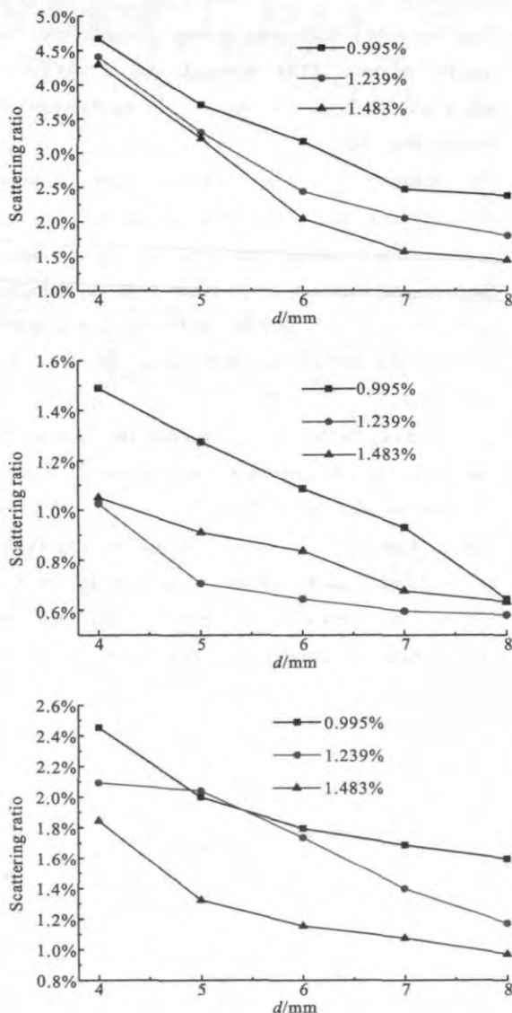
图 7 琼脂糖凝胶激光散射率(a)440 nm;(b)532 nm;(c)650 nm
