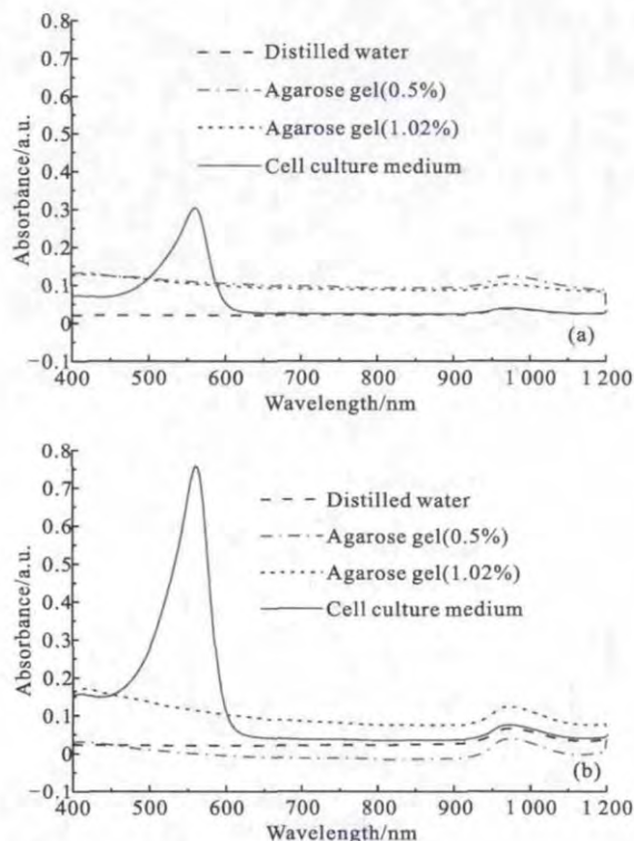
图 4 琼脂糖凝胶与细胞培养液 FOSS 透射近红外光谱(400~1 100 nm)(a)样品厚度 1 mm;(b)样品厚度 2 mm
