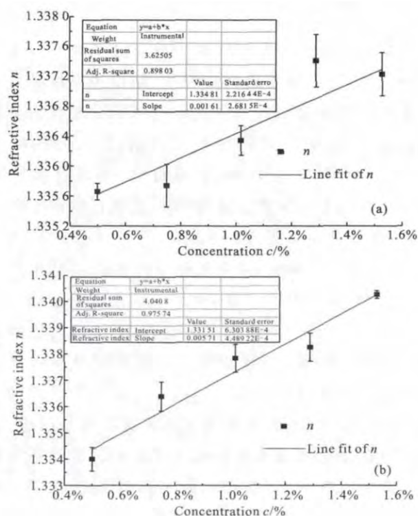
图 2 琼脂糖溶液折射率
