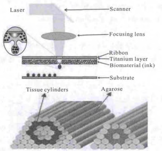
图 1 琼脂糖凝胶作为基质材料及生物支架
