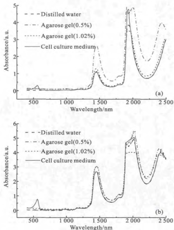
图 3 蒸馏水、琼脂糖凝胶(0.5% 浓度和 1.02% 浓度)和细胞培养液 FOSS 透射光谱(a)样品厚度 1 mm;(b)样品厚度 2 mm
