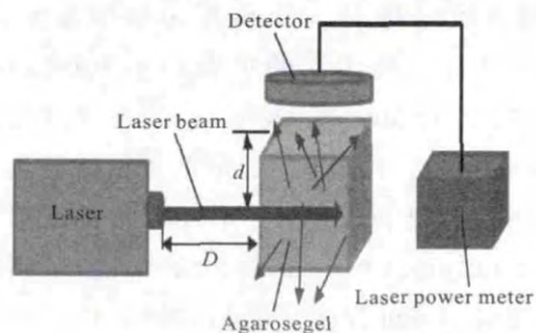
图 6 琼脂糖凝胶激光散射实验示意图
