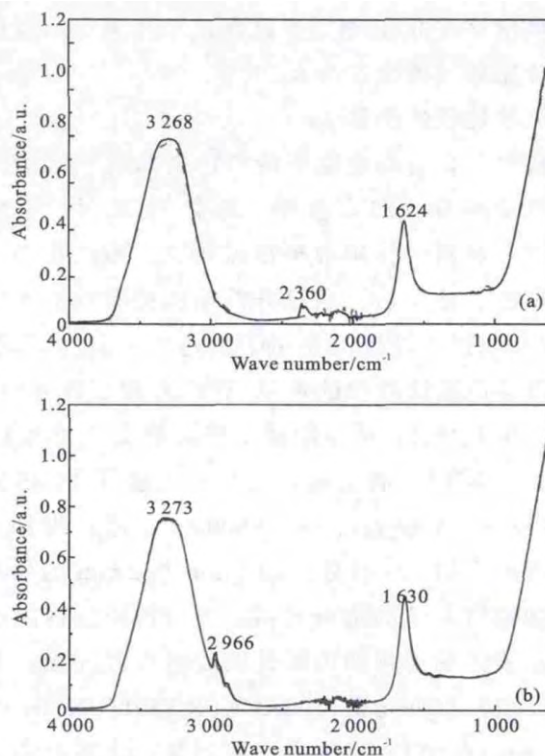
图 5 琼脂糖凝胶 FTIR-ATR 光谱(a);细胞培养液 FTIR-ATR 光谱(b)
