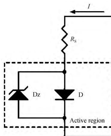
图 1 半导体激光器简化等效电路
