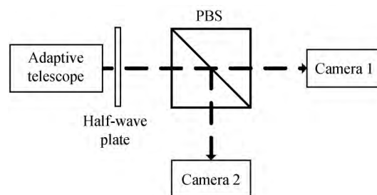
图8 改进偏振成像方案示意图
