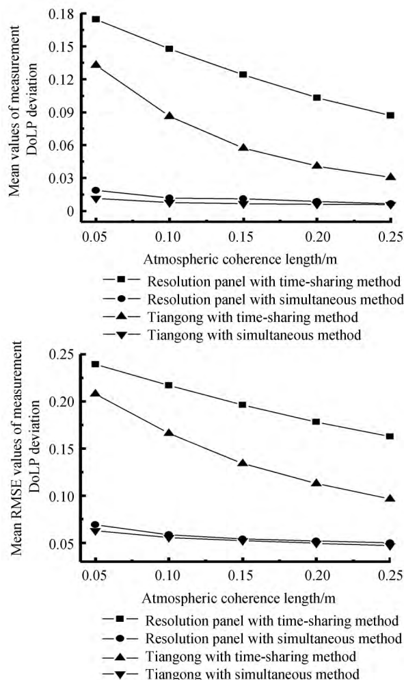
图 6 偏振度探测偏差随大气相干长度变化
