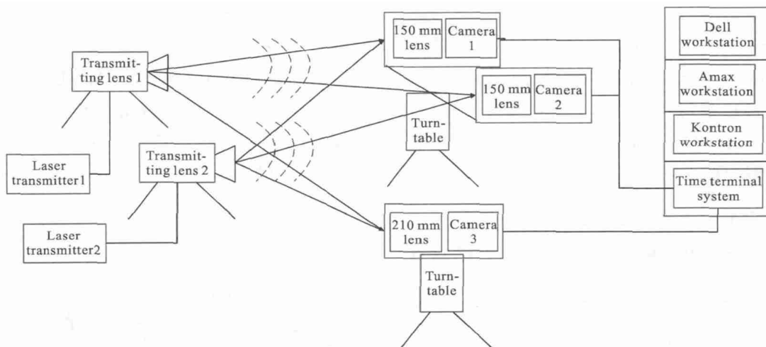
图 3 实验平台框图
