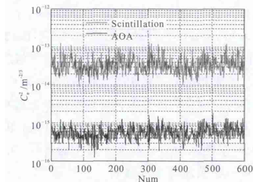
图 6 等功率单发单收结果
