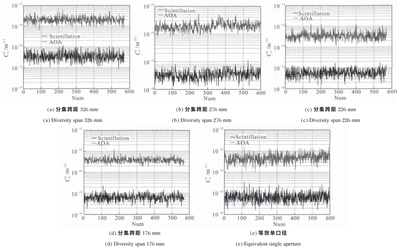
图 8 分集接收结果
