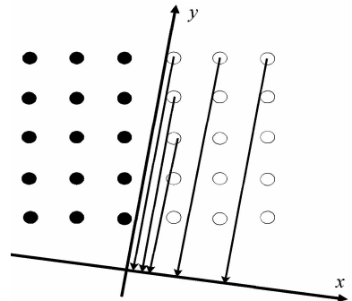
图 2 倾斜刃边法投影示意图
