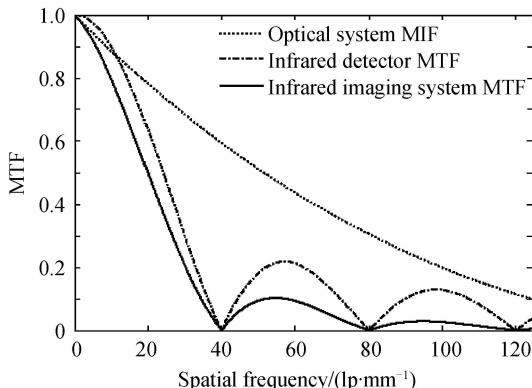
图 8 红外成像系统的 MTF 曲线
