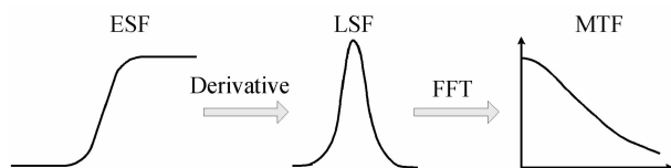
图 1 倾斜刃边法测试 MTF 原理
