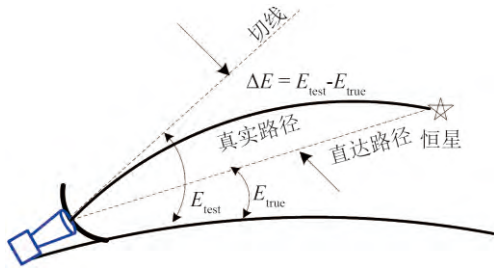
图 4 船载星敏器蒙气差修正
