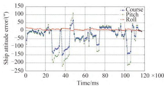
图8 星敏感器 A_2 测量船体姿态误差
