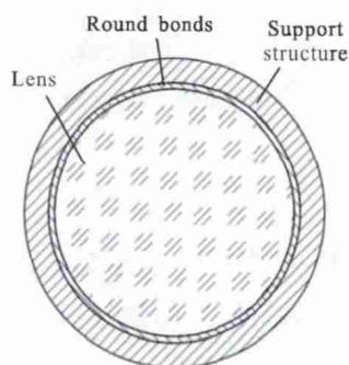
图 2 一般透镜组件装配结构示意图
