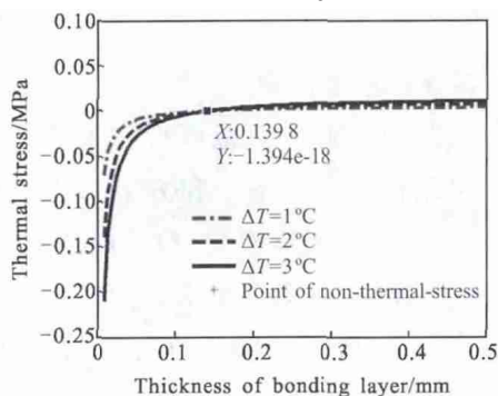
图 4 \Delta T 为 1 °C、2 °C、3 °C 时, 热应力随胶层厚度变化曲线
