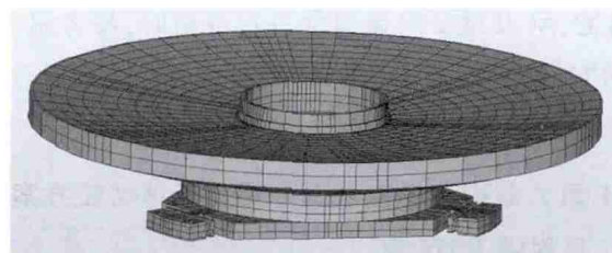
(a) 组件的有限元模型
