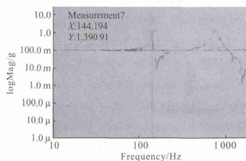
图 10 X 向随机试验前的 0.1 g 扫频曲线
