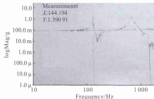
图 11 X 向随机试验后的 0.1 g 扫频曲线
