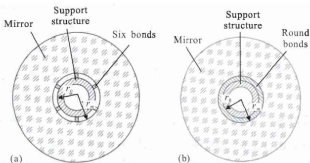
图 3 方案一和方案二
