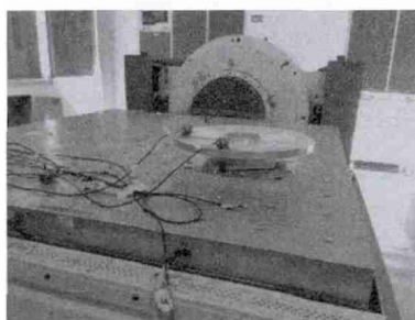
图 9 反射镜组件振动试验现场
