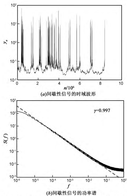
图1 采用SDEs生成的间歇性信号和该信号的功率谱密度
