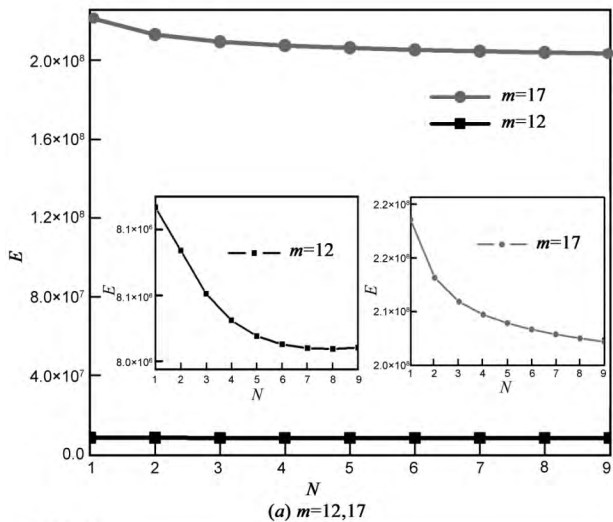
图2 小波系数方差与尺度的关系
