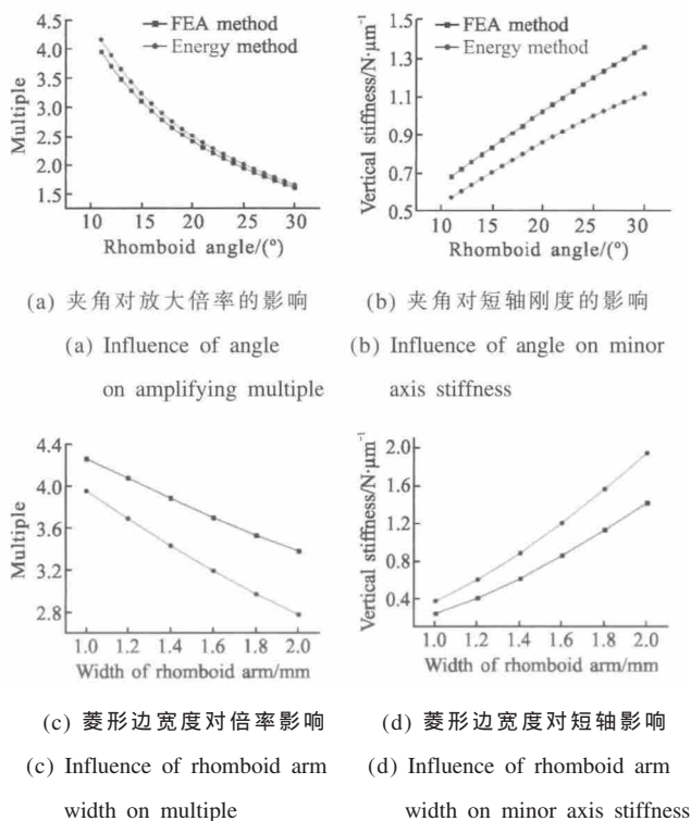
图 3 关键参数对菱形结构性能的影响
