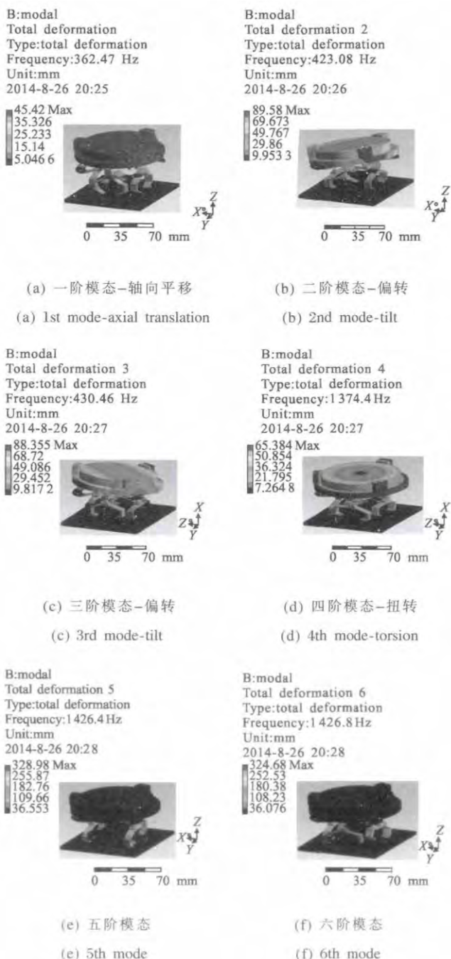
图 6 FSM 系统模态有限元分析
