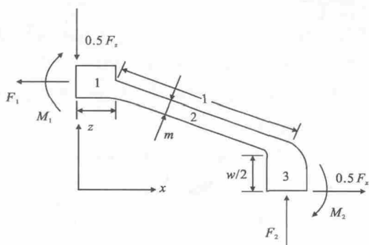
图 2 菱形结构受力分析
