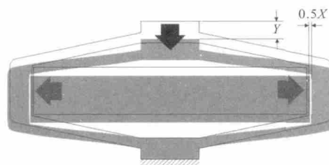
图 1 菱形结构位移放大原理示意图
