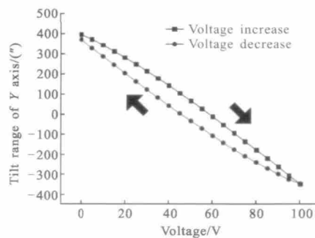
图 8 快速反射镜偏摆范围测试结果
